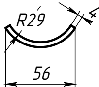
Поз.3 (Подушка)
